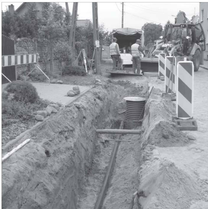
Budowa kanalizacji w Dąbrówce Wlkp.
